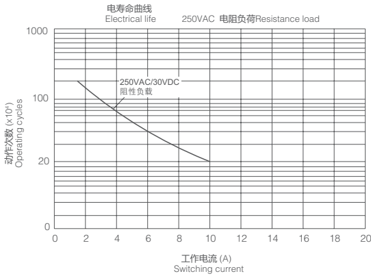
2CO 电寿命曲线图
