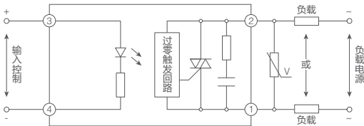
直流输入型
