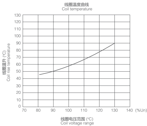
2CO/3CO/4CO 线圈温度曲线图
