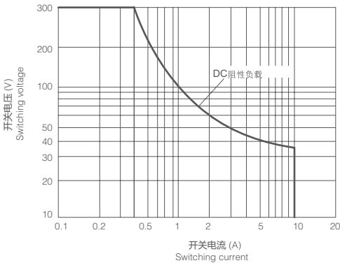
2CO 最大功率切换图
