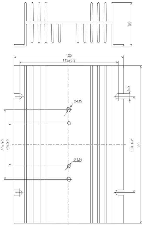
AOCR-R4
