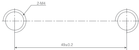
安装孔尺寸图
