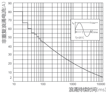
浪涌持续时间曲线图（负载电流 2A）
