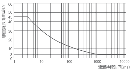
浪涌持续时间曲线图 (负载电流为 3A, 负载电压为 DC48V)
