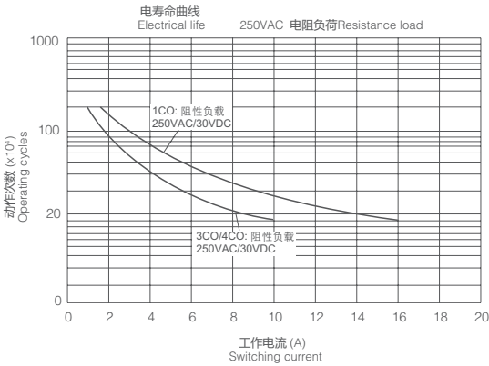
1CO/3CO/4CO 电寿命曲线图
