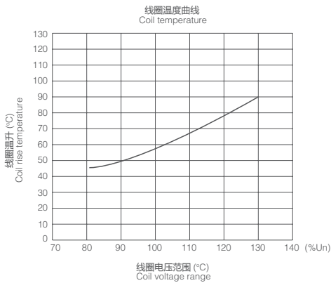
1CO 线圈温度曲线图
