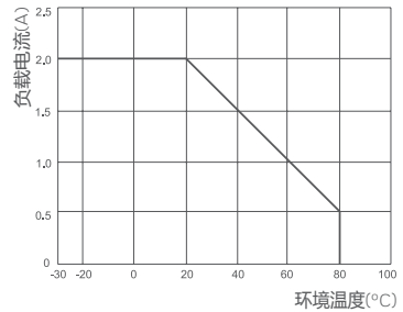
最大负载电流与环境温度曲线图（2A）
