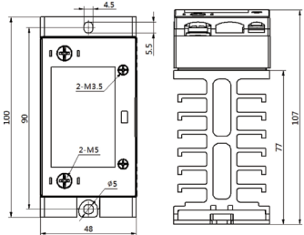
OCR-D 单相交流固态继电器尺寸图
