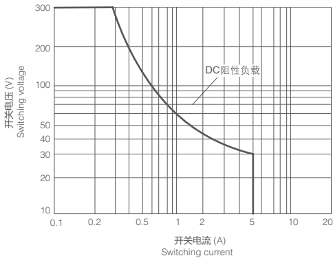
4CO 最大功率切换图
