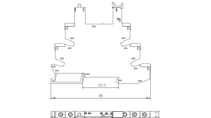
安装尺寸图 PSR-1C- *-E
