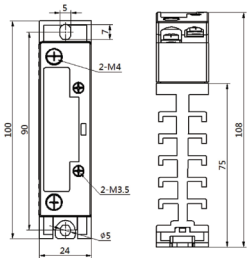
OCR-D 单相交流固态继电器尺寸图
