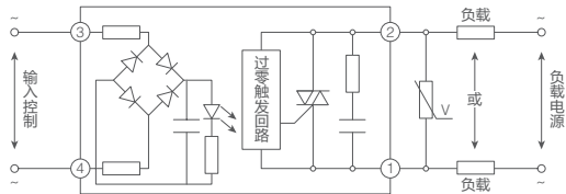
交流输入型
