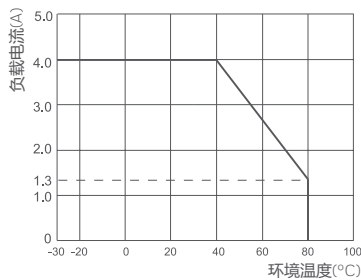
最大负载电流与环境温度曲线图 (4A)
