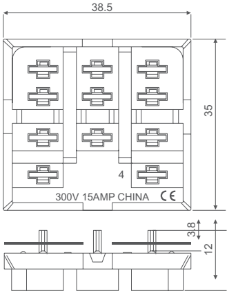
底座尺寸图 PHRM-P
