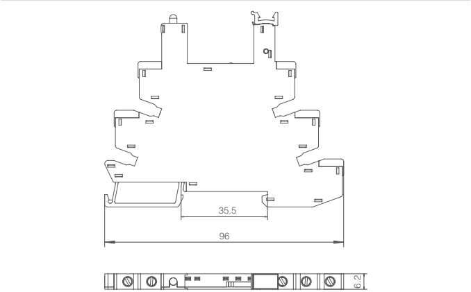
安装尺寸图 PSR-1C- *-E
