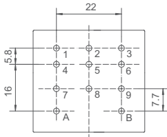
底座接线图 PHRM-P
