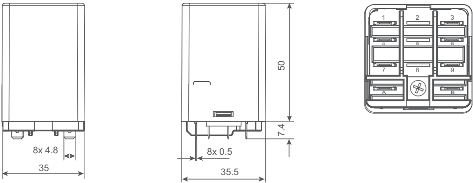
继电器接线图
