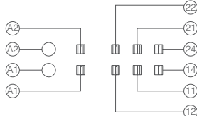
端子配置内部接线图 PCR-2C-E
