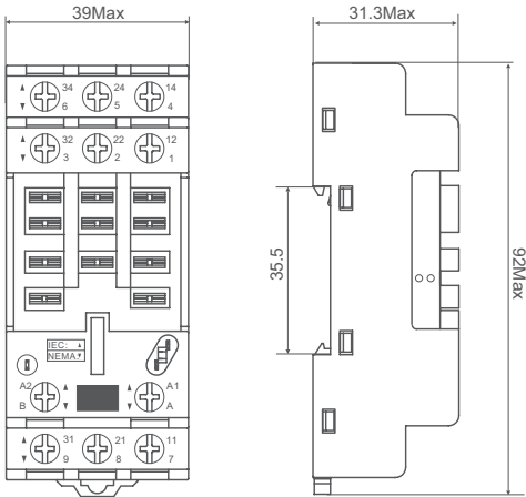
底座接线图 PHRM-E
