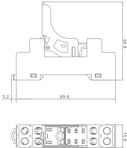
PCR-2C-T
