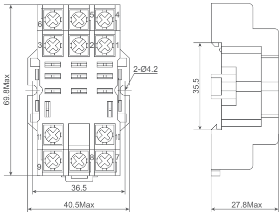
PHR-3C-E
