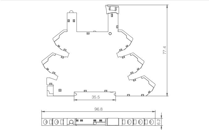
安装尺寸图 PSR-1C- *-S
