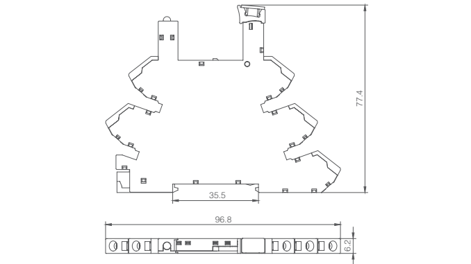
安装尺寸图 PSR-1C- *-S
