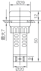
面板开孔: Ø22(Ø25)
