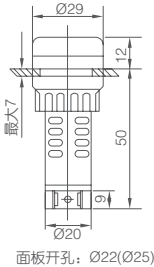
面板开孔: Ø22(Ø25)
