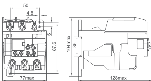
HRS-C-...-P 独立式安装 (配合背包 HAS-RC-P)
