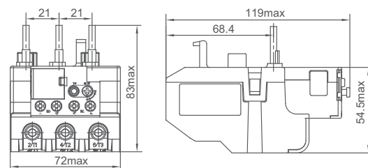
HRS-C-...-P 组合式安装 (配合相应 HCS-...-P 接触器)
