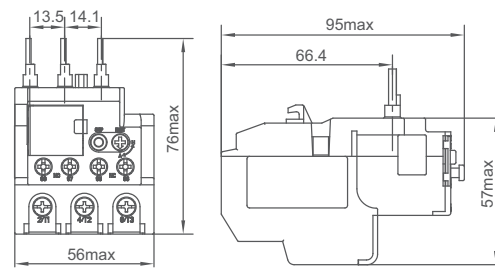
HRS-B-...-P 组合式安装 (配合相应 HCS-...-P 接触器)
