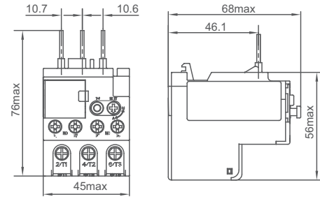
HRS-A-...-P 组合式安装 (配合相应 HCS-...-P 接触器)
