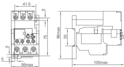
HRS-B-...-P 独立式安装 (配合背包 HAS-RB-P)
